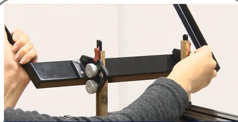
5. ガラスフレームを上から差し込み、 適切な高さで両脇のねじを締めます。
