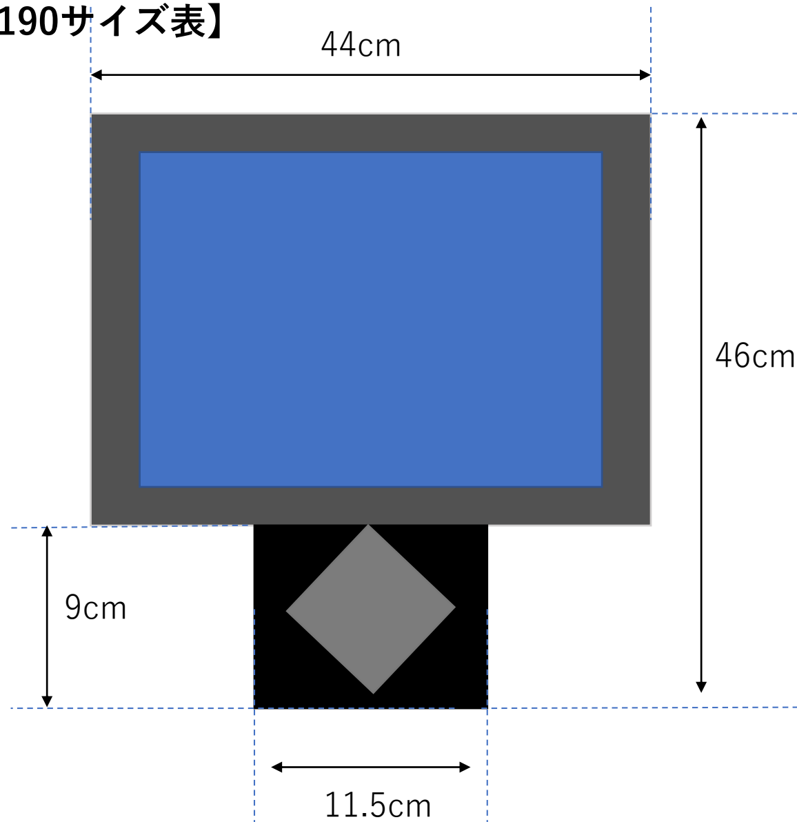
【上面図】
